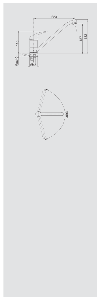
jasmín 515 361 tlaková
